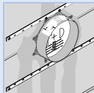
Szerelés a falban, szerelősinék segítségével
