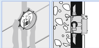
Szerelés közvetlenül a falba süllyesztve
