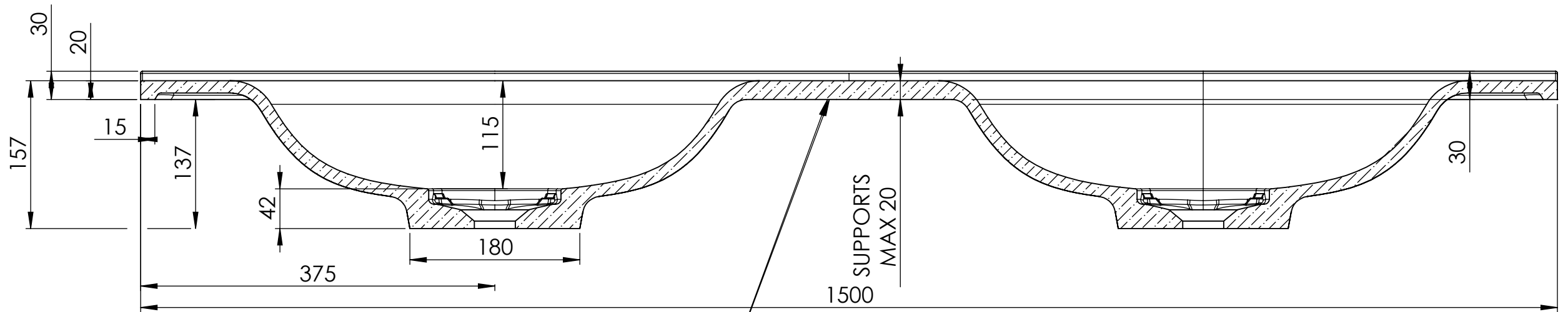
A-A (1 : 5)
