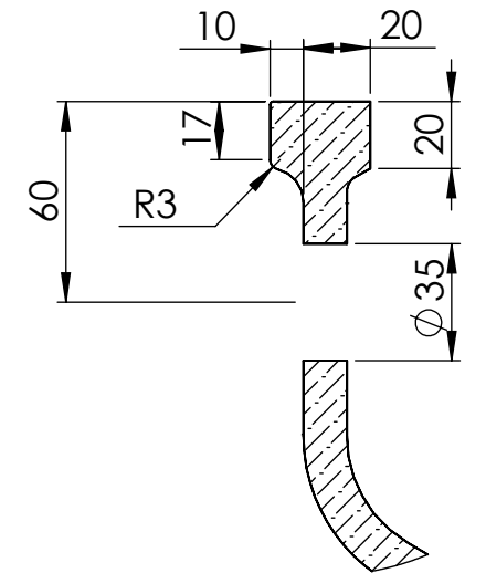
C (2 : 5)
