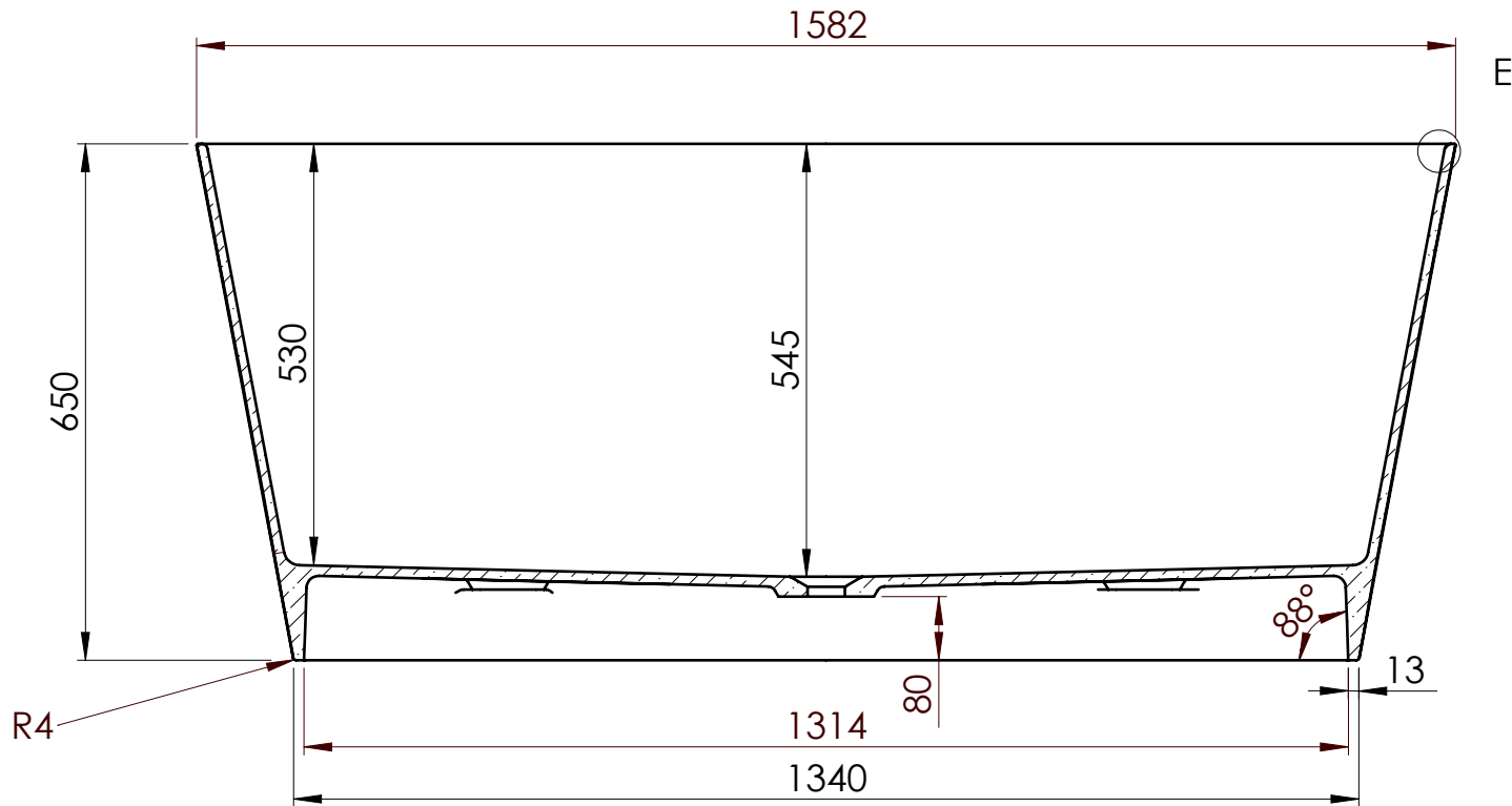
A-A (1 : 10)
