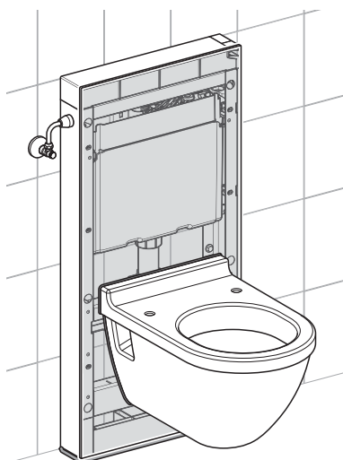
Fali WC-kerámiához
