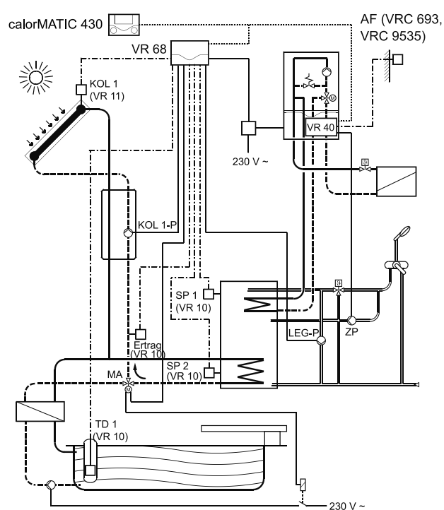
1 fűtési kör calorMATIC 430 szabályozóval, VR 68 modulal, szolár melegvíztárolóval és medencével
